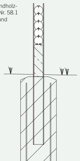
Schnittzeichnung: Fundament mit HEA-Träger, Betonteil und Rundhölzern
