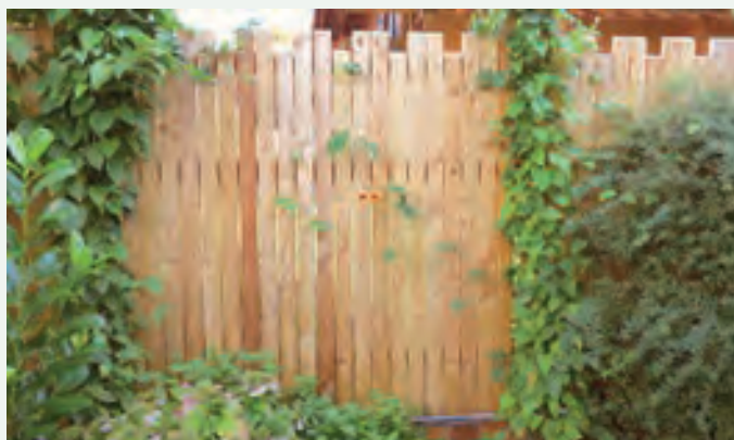
Sichtschutzzaun mit höhenversetzten Hobellatten 25 x 65 mm.
