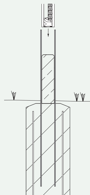
Schnittzeichnung Fundament mit HEA-Träger und Betonteil
