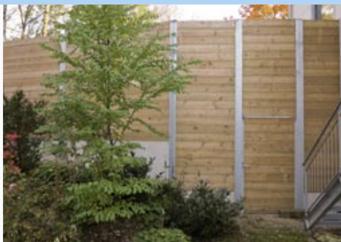
Lärmschutzwand Nr. 58.5, ca. 4 m hoch mit Bohlen 77 x 160 mm und Betonteil. Wandanschluss mit U-Träger und Lärmschutztüre auf Stahlrahmen
