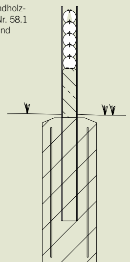
Schnittzeichnung: Fundament mit HEA-Träger, Betonteil und Rundhölzern
