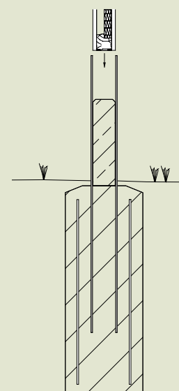
Schnittzeichnung Fundament mit HEA-Träger und Betonteil
