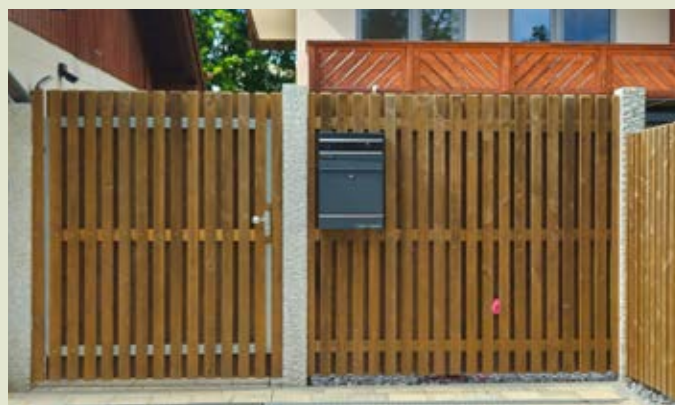
Sichtschutzwand mit Eisentor, Fichte braun kesseldruckimprägniert, mit beidseitig versetzt angebrachten Hobellatten 25 x 65 mm, oben schräg.
