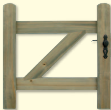
Geschraubter Torrahmen ohne Füllung
