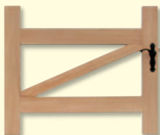
Verzapfter H-Rahmen ohne Füllung
