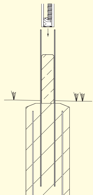
Schnittzeichnung Fundament mit HEA-Träger und Betonteil
