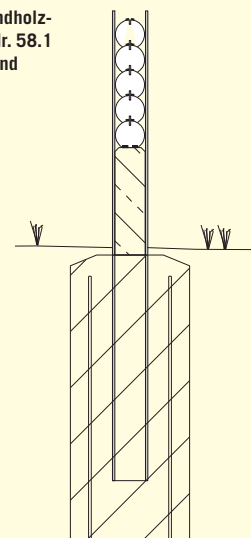
Schnittzeichnung: Fundament mit HEA-Träger, Betonteil und Rundhölzern
